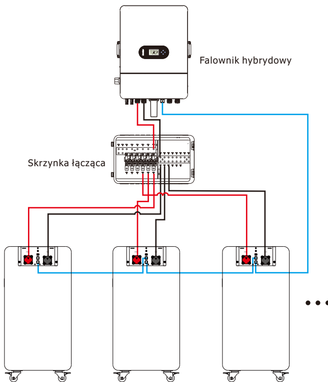
Rysunek 4-1 Równoległe połączenie trzech zestawów baterii
