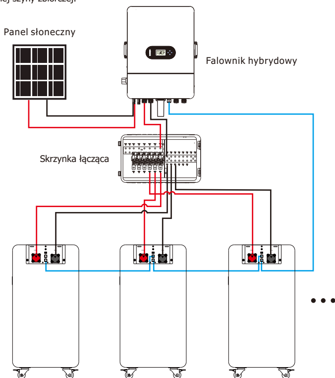
Rysunek 3-2 Schemat połączenia wielu baterii w układzie równoległym
