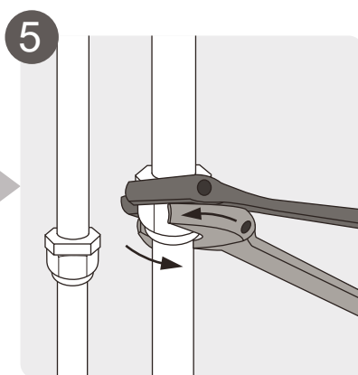
Podłącz rurociągi
